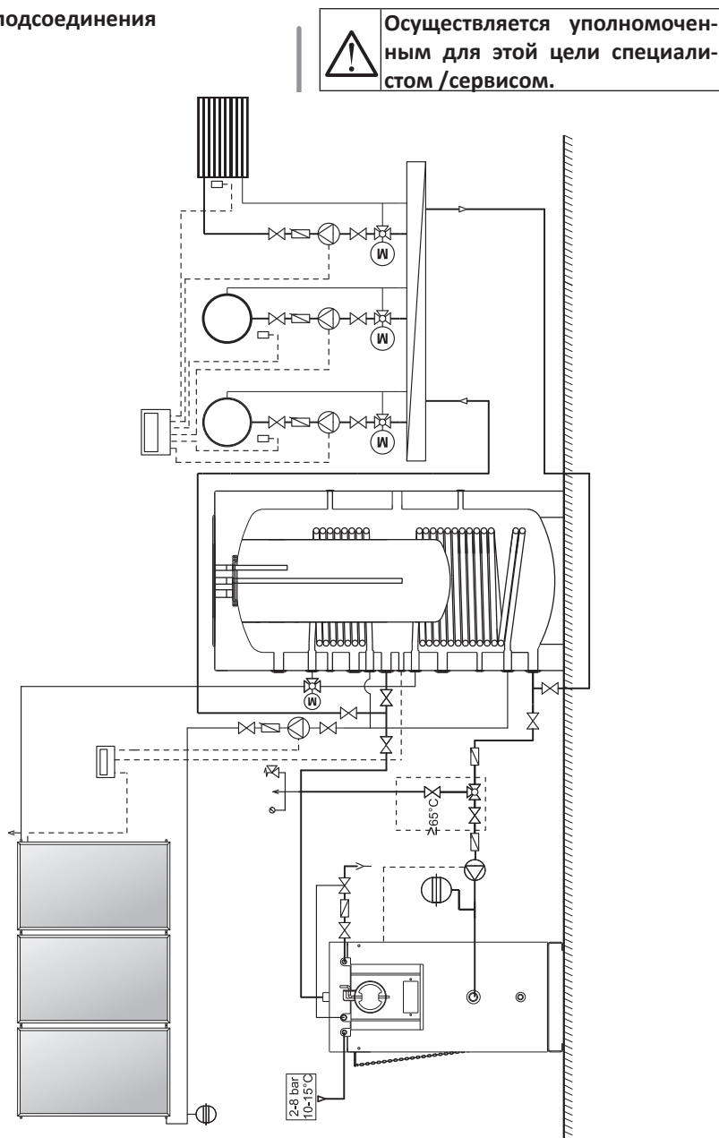
Схема 24. Подсоединение солнечной панели-коллектора PK к котлу WBS, комбинированному бойлеру KSC2 и трехдорожному вентилю
