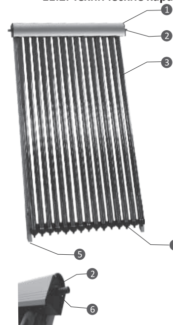
Схема 29. Элементы вакуумно-трубного коллектора VTC
